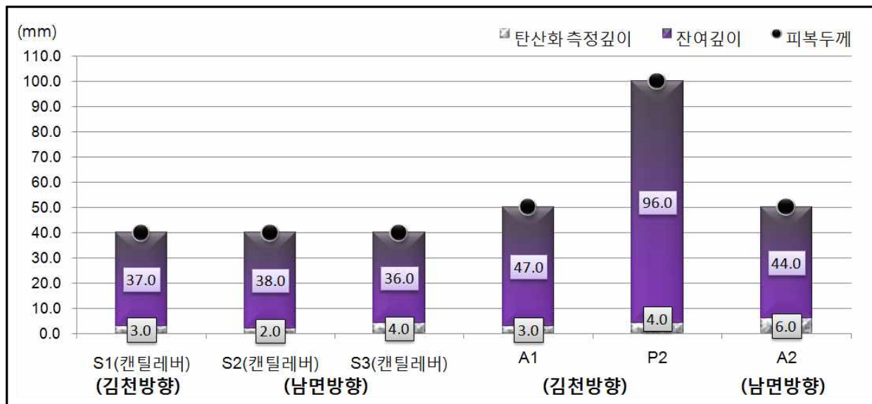
【그림 4.3】 탄산화 진행깊이 및 잔여깊이 측정결과
